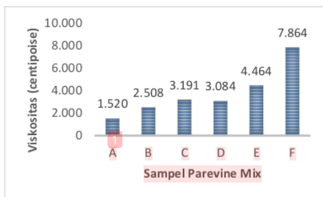
Gambar 1. Viskositas parevine mix
